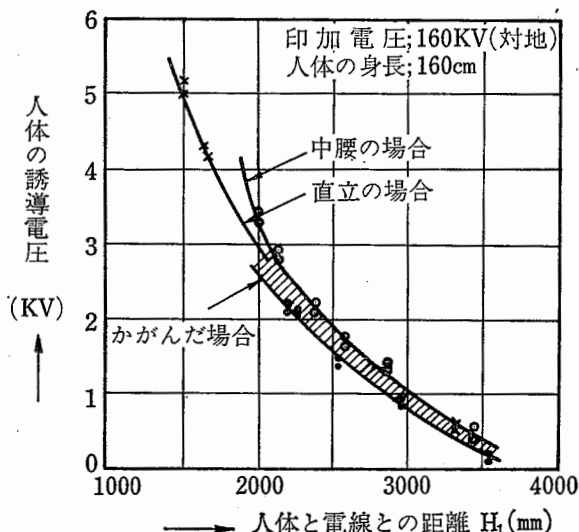
図 6-9 線路からの距離と人体の誘導電圧の関係
