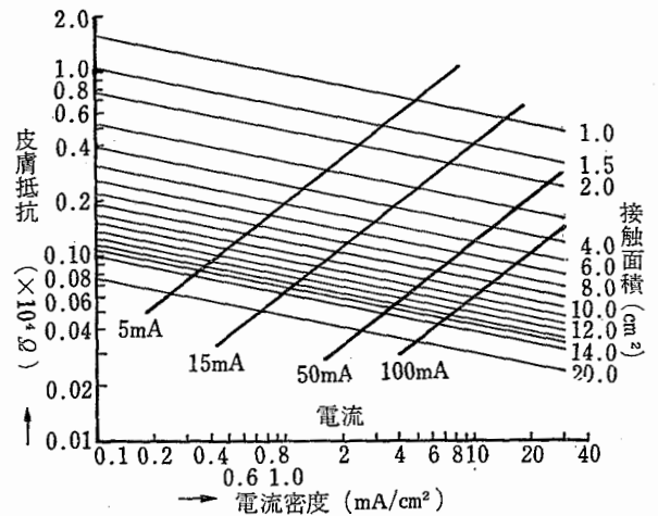
図 3-2 湿った手における皮膚抵抗と電流密度、接触面積との関係
