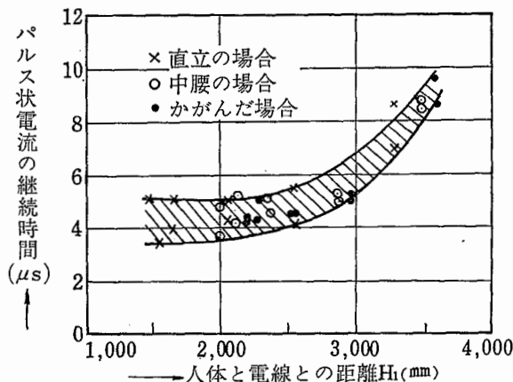
図 6-16 線路からの距離と人体のパルス電流継続時間の関係（指先で接触したとき）
