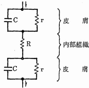
図 3-6 人体の電気的等価回路
