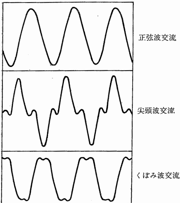
〔資料 2〕 Dalziel が可随電流の実験に用いた交流波形のオシログラム
