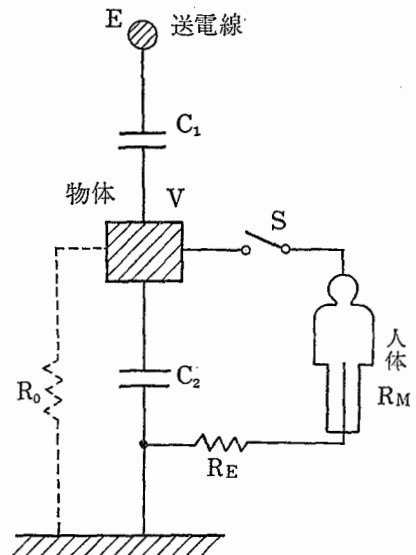
C_1 : 送電線と物体間の静電容量 C_2 : 物体と大地間の静電容量 R_M : 人体抵抗 R_E : 人体と大地の接触抵抗 R_0 : 物体の対地絶縁抵抗 E : 送電線の対地電圧 V : 静電誘導電圧
