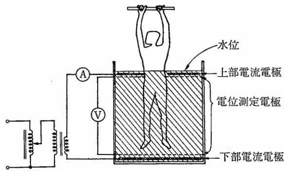
図 5-3 足の自由を失なう電界測定の実験回路 電界中では水中にいる人の泳ぐ能力を失なわせるのでこの電界が実際の致死レベルであると考えられる。
