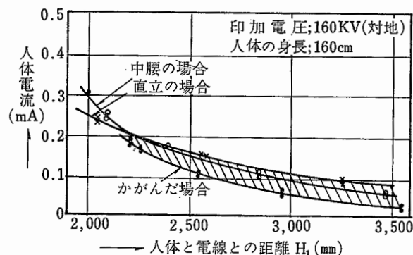
図 6-10 線路からの距離と人体電流との関係
