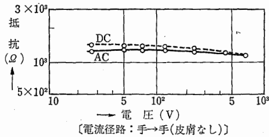
図 3-7 人体の内部抵抗
