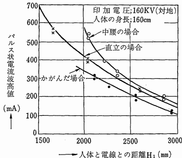
図 6-15 線路からの距離と人体のパルス電流波高値の関係（指先で接触したとき）
