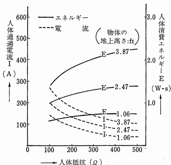
図 6-12 開閉サージ ( 1 \times 2,000 \mu s ) に対する人体抵抗, 人体通過電流, エネルギーの関係
