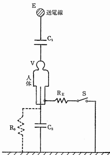
C_1 : 送電線と人体間の静電容量 C_2 : 人体と大地間の静電容量 R_E : 人体と大地との接触抵抗 R_0 : 人体の対地絶縁抵抗 E : 送電線の対地電圧 V : 静電誘導電圧
