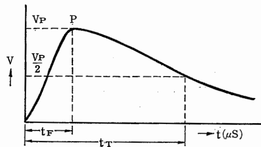
〔資料 10〕 衝撃電圧波形の表わし方
