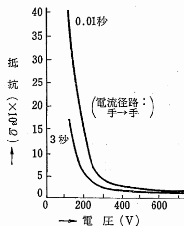
図 3-5 抵抗値の時間的变化
