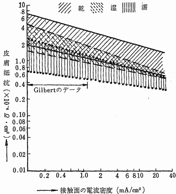
図 3-1 皮膚の湿り度合による皮膚抵抗の変化
