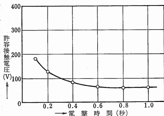
図 4-1 通電時間と許容接触電圧 (VDE 0141/2.64による)
