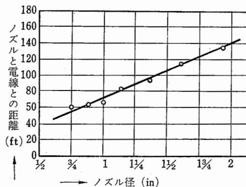
図 7-6 ノズルの直径とノズル-電線間の距離
