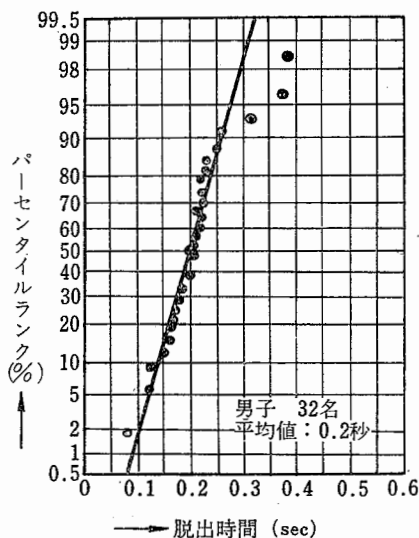
図 2-7 可随電流に対する脱出時間 (60Hz)
