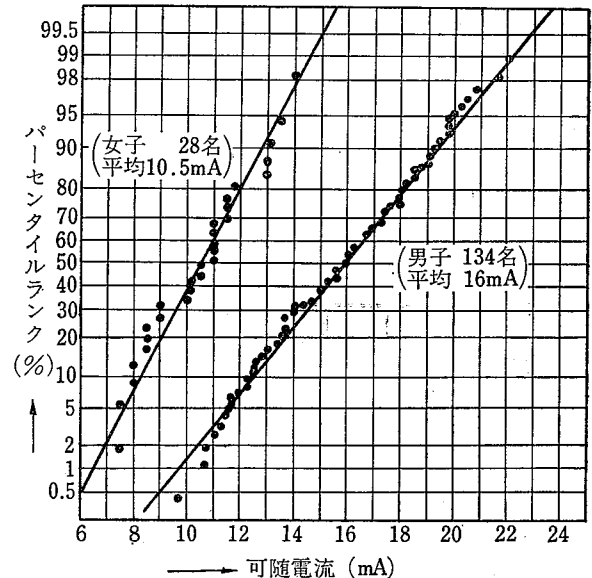
図 2-4 60Hz 正弦波交流による可随電流
