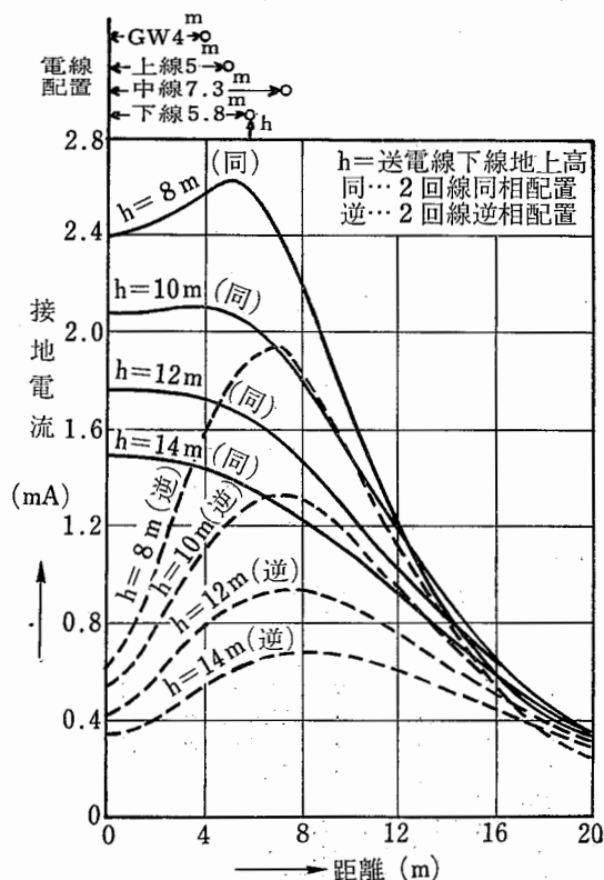
図 6-5 275kV 2 回線送電線下の接地電流 (モデル：大型バス)
