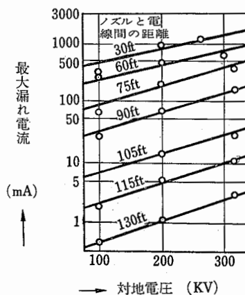
図 7-3 対地電圧と漏れ電流
