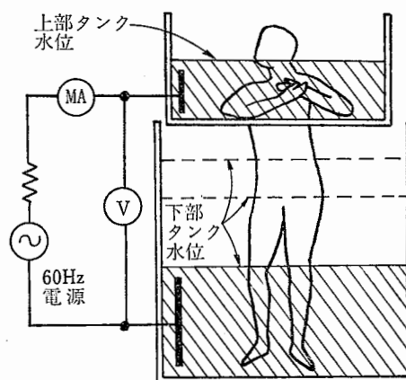
図 5-2 電界測定の試験回路
