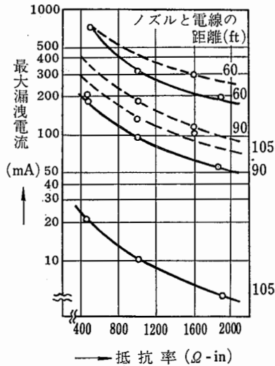
図 7-4 水の抵抗率と漏れ電流 ——交流 .....直流
