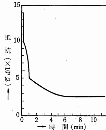
図 3-4 印加時間による抵抗の変化
