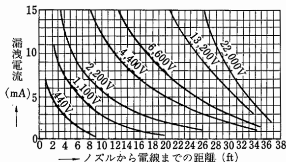
図 7-1 注水距離と漏れ電流
