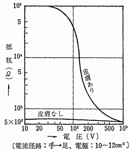
図 3-3 印加電圧による人体抵抗の変化
