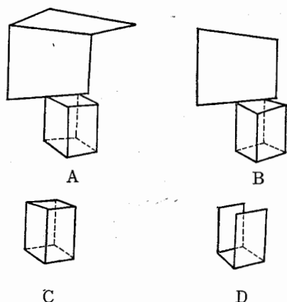
A: 背後の壁と頭上のおおいをもつ完全なバスケットしゃへい B: 背後の壁をもつ完全なバスケットしゃへい C: 完全なバスケットしゃへい D: 部分的なバスケットしゃへい
