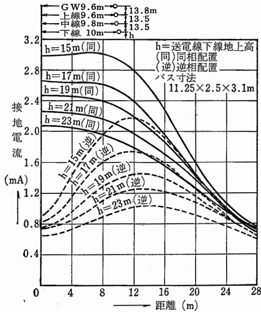
図 6-6 520 kV 2 回線送電線下の接地電流 (モデル：大型バス)
