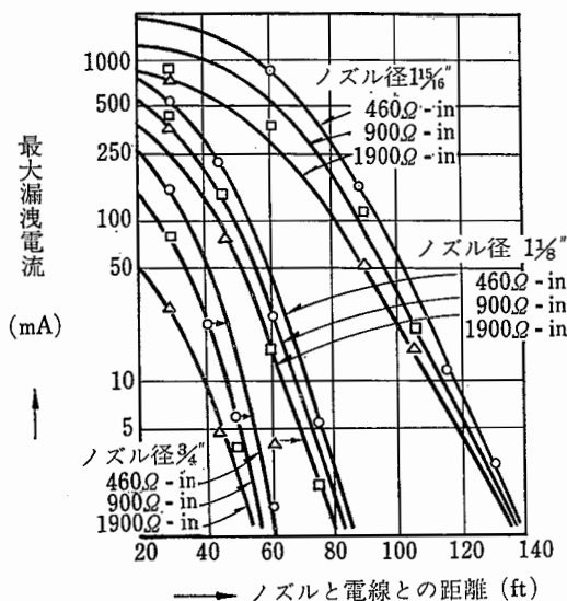
図 7-2 ノズル-電線間の距離と漏れ電流
