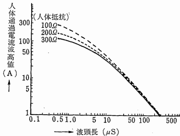
図 6-14 サージの波頭長（波尾長は 2,000\mu\text{s} で一定）と人体通過ピーク電流の関係
