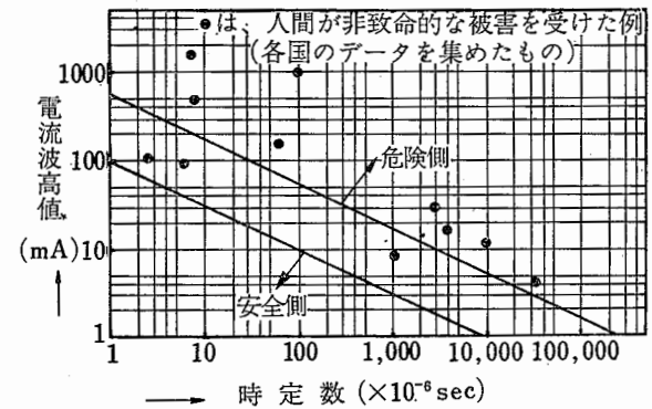
図 6-17 インパルス電流の理論的危険限界
