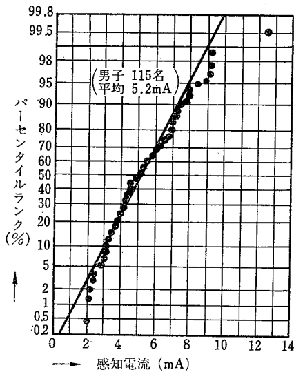
図 2-3 直流による感知電流
