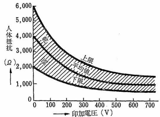
図 3-8 人体抵抗範囲
