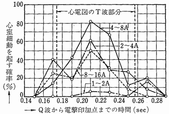
図 2-19 電撃印加位相と心室細動を起こす確率との関係 (羊, 60Hz, 通電時間 0.03 秒)
