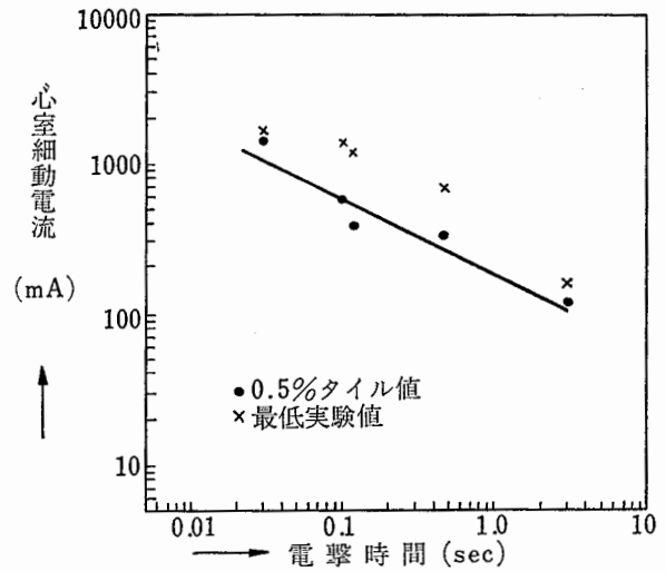
〔資料 4〕 通電時間と心室細動電流 (犬) (東京大学医学部における実験データ)
