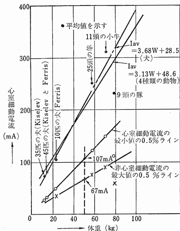
図 2-13 各種の動物に対する心室細動電流と体重の関係 (通電時間3秒)
