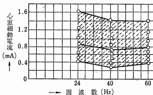
図 2-16 正弦波交流における周波数と心室細動電流との関係 (犬, 通電時間 2 秒)
