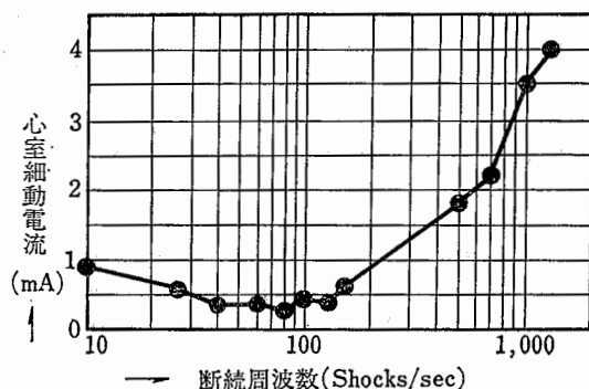
図 2-15 矩形波断続電流の周波数と心室細動電流 (犬, 通電時間 2 秒)
