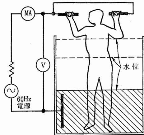
図 5-1 電位測定の実験回路
