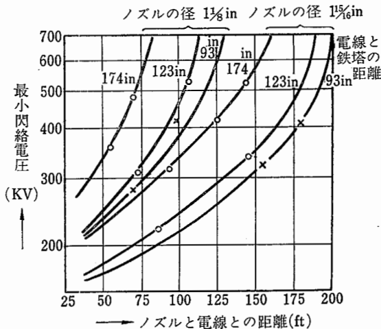
図 7-5 直流でのフラッシュオーバー電圧
