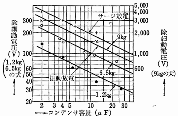
放電形式による除細動電圧の変化
