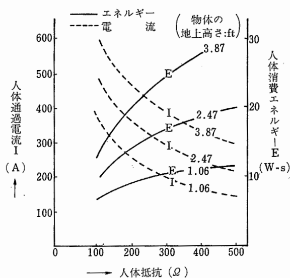
図 6-13 雷インパルス ( 1.5 \times 40 \mu s ) に対する人体抵抗, 人体通過電流, エネルギーの関係
