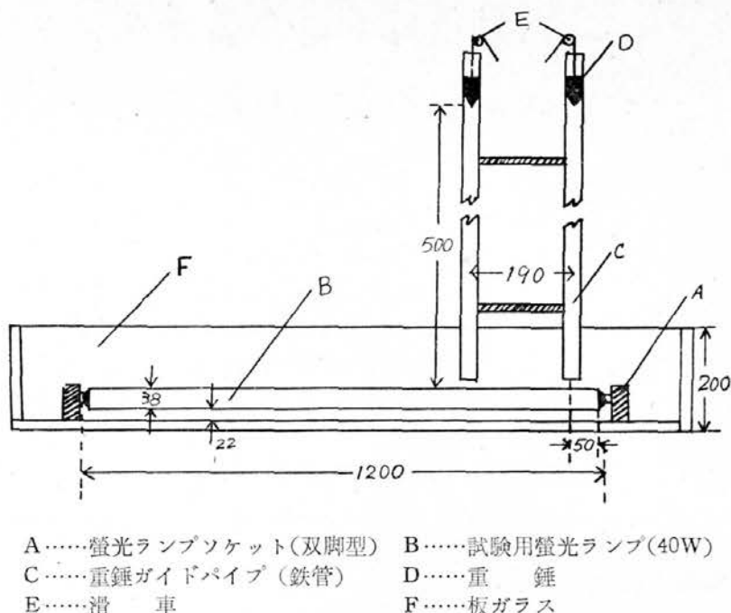
図5 蛍光ランプの破壊試験装置(単位mm)
