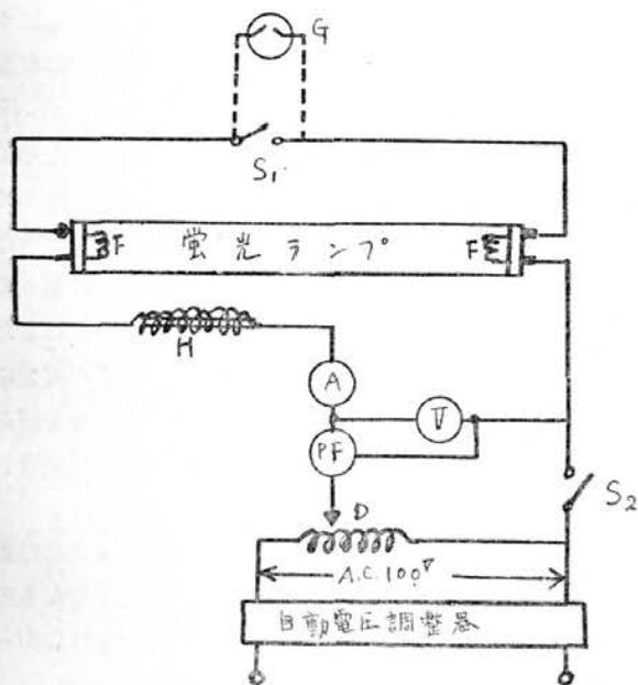
図 8 蛍光ランプ破壊試験回路接続図
