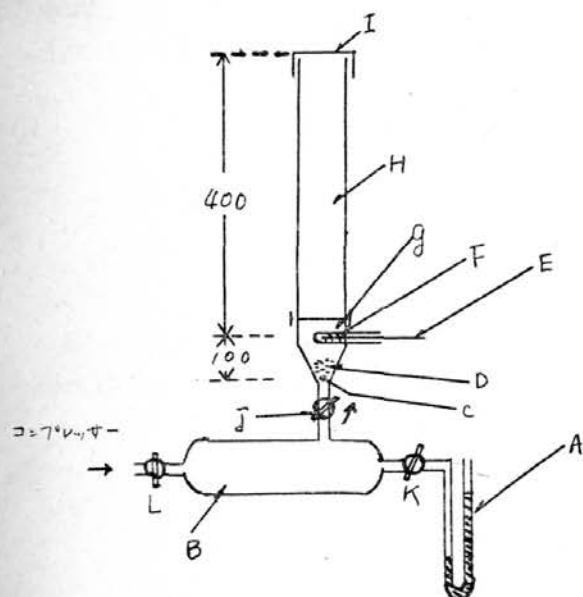
図 1 粉塵爆発試験装置 (単位 mm)
