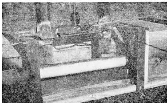
図 9 蛍光ランプ破壊前の状態
