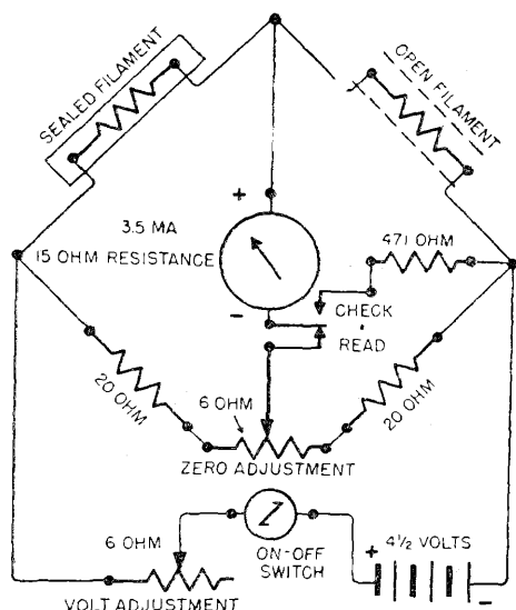
図 7 燃焼式爆発計配線図
