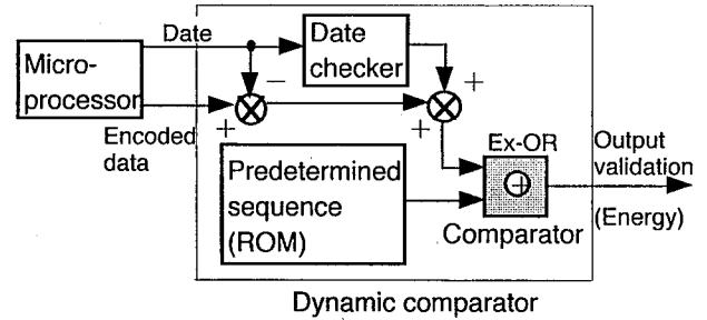
Fig. 4 Principle of code checking by dynamic comparator. ダイナミックコンパレータによる符号チェックの原理
