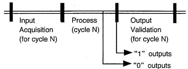
Fig. 6 Program sequence for output check cycle. 出力チェックサイクルのためのプログラムシーケンス
