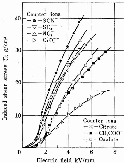
Fig. 6 Effects of counter ion (inorganic acid ions and organic acid ion) 対立イオンによる影響(無機酸イオンおよび有機酸イオン)
