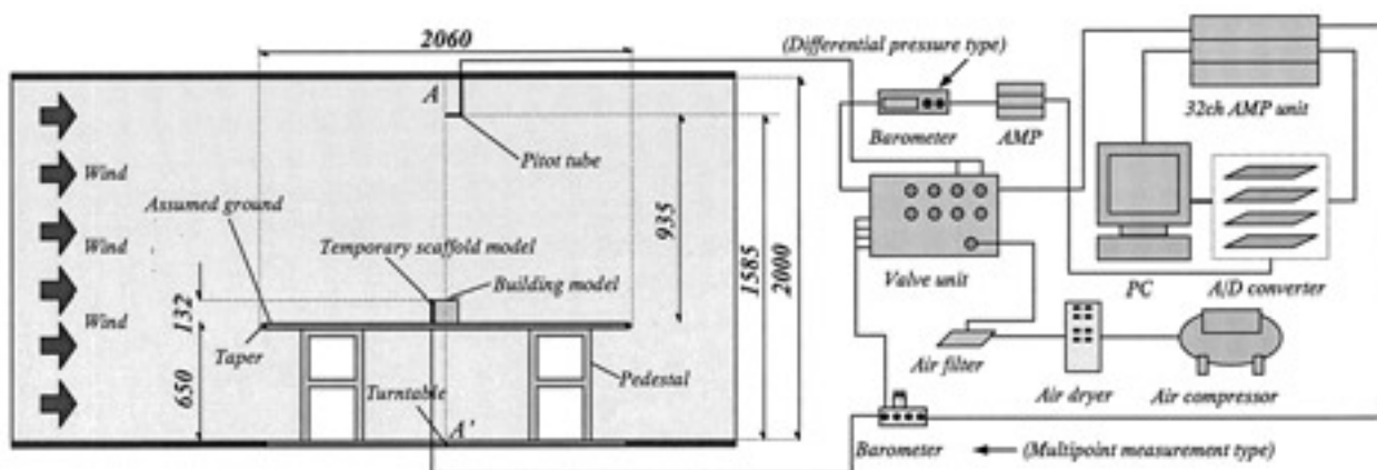
Fig. 3 Experimental configuration (unit: mm) 実験システムの概念図
