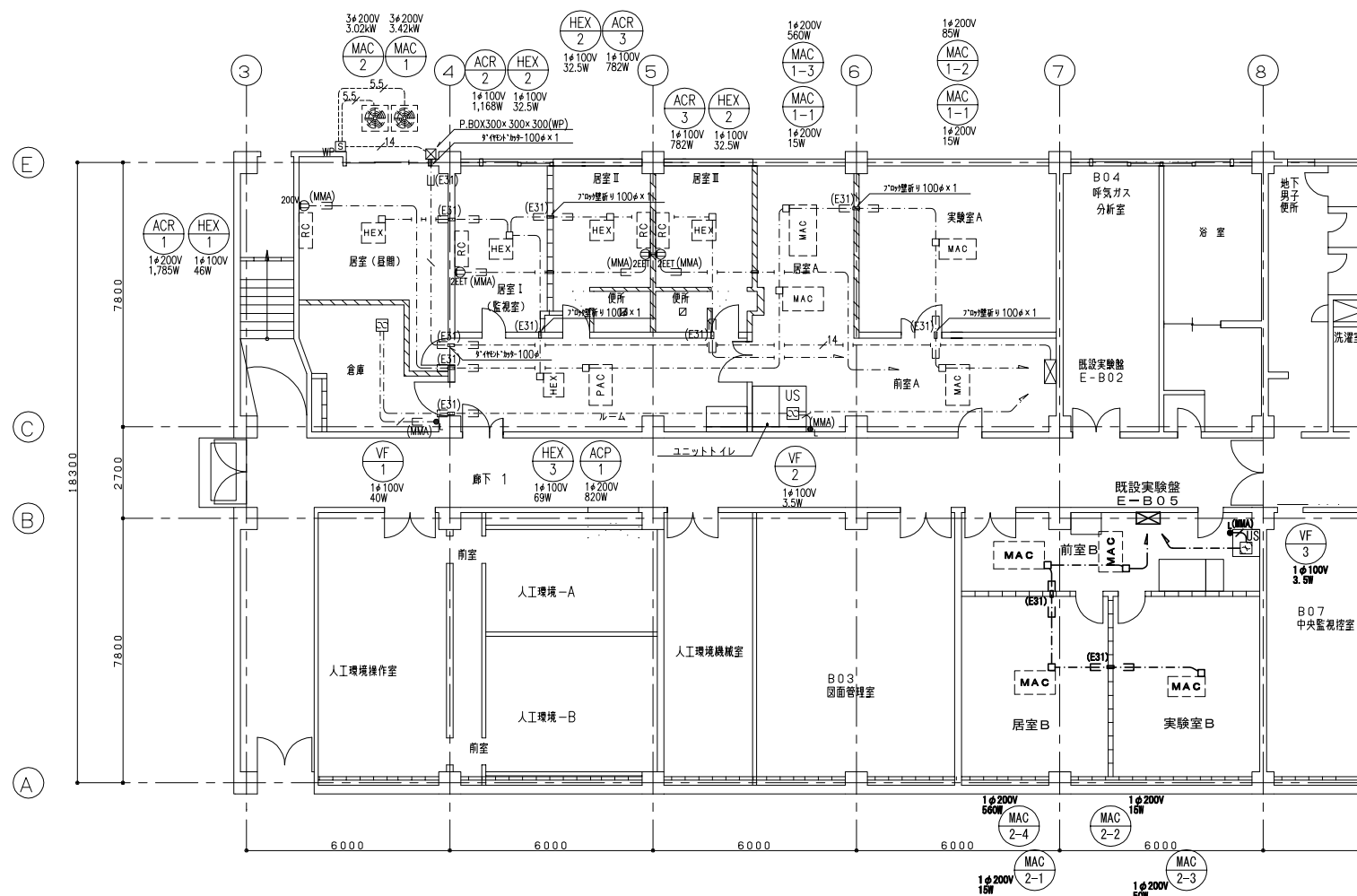
改設 研究本館 電気設備 B1階空調電源設備平面図 S=1/100
