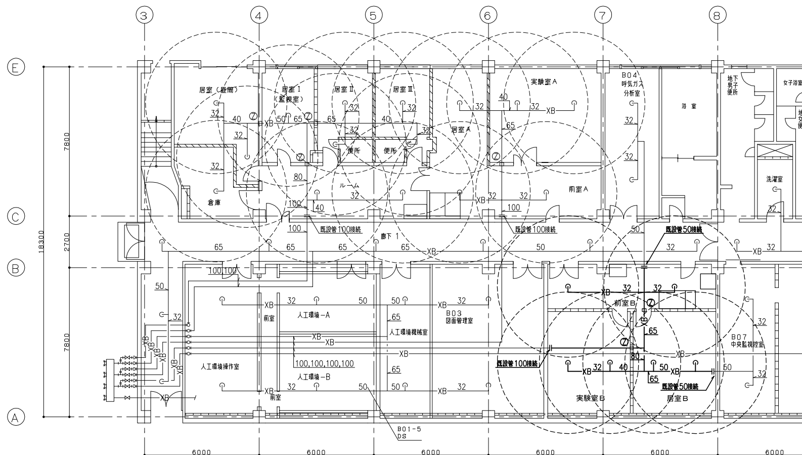
改修 研究本館 消火設備 B1階平面図 S=1/100
