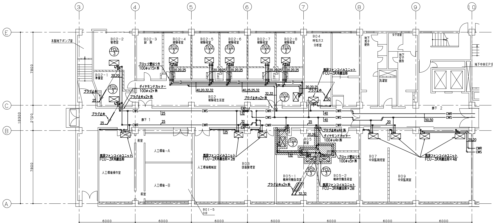
撤去 研究本館 空調設備 B1階空調配管平面図 S=1/100
