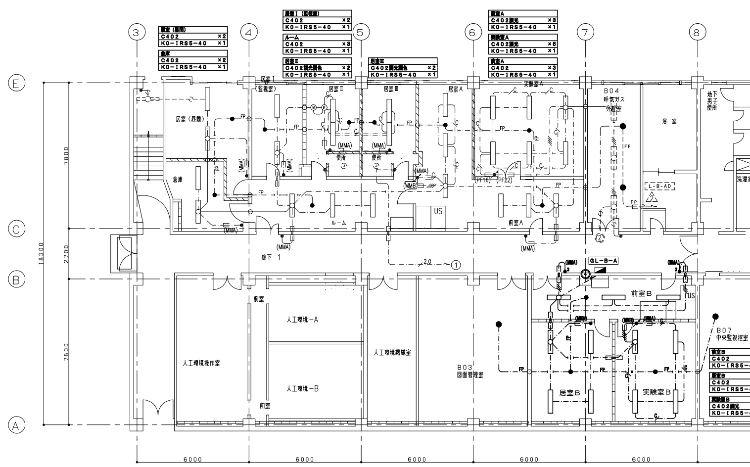
改設 研究本館 電気設備 B1階電灯設備平面図 S=1/100
