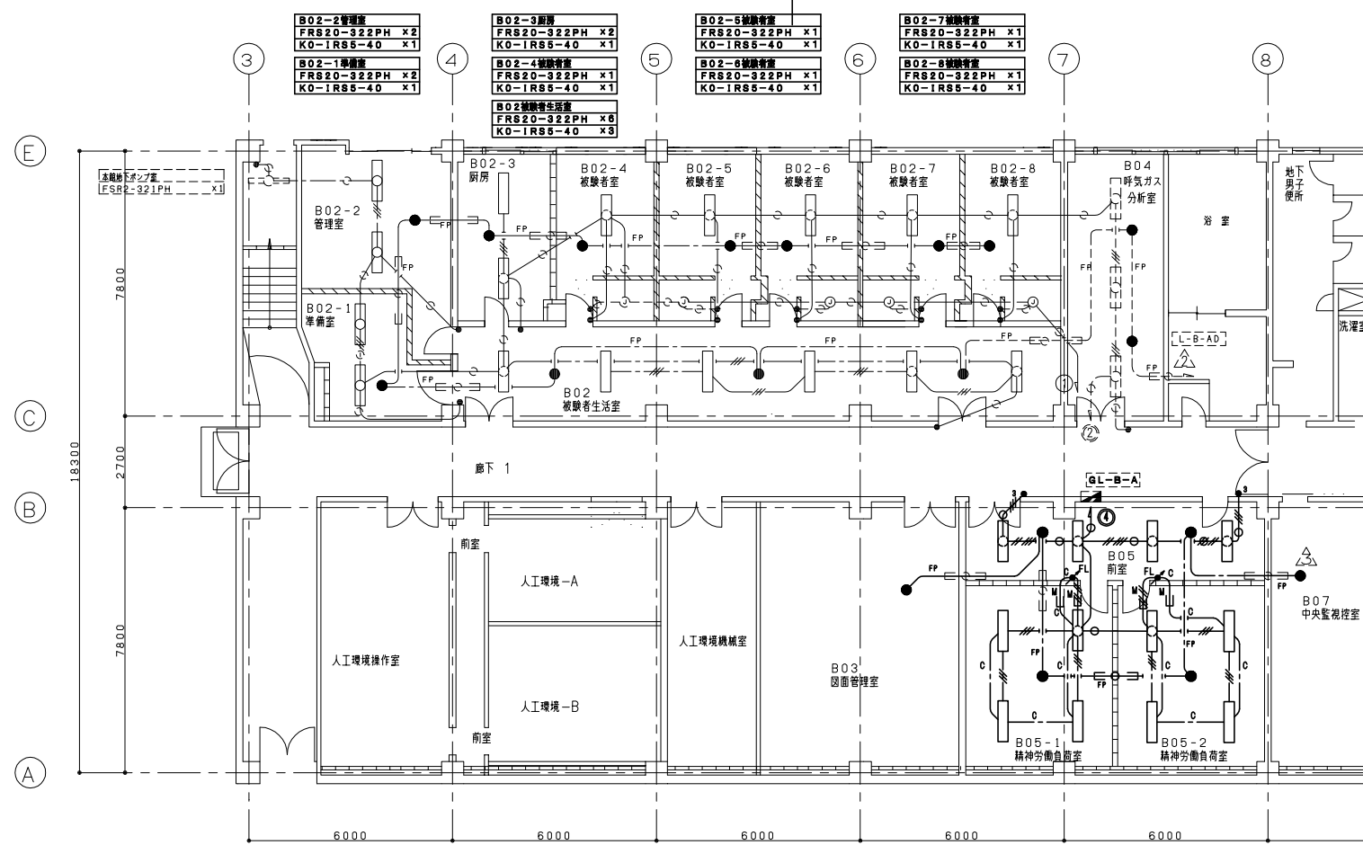
撤去 研究本館 電気設備 B1階電灯設備平面図 S=1/100
