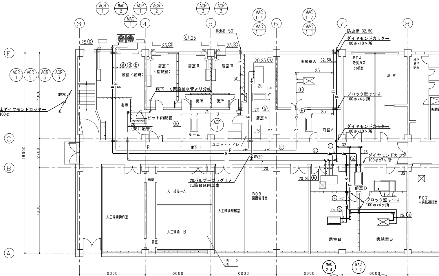
改設 研究本館 空調設備 B1階ダクト平面図 S=1/100
