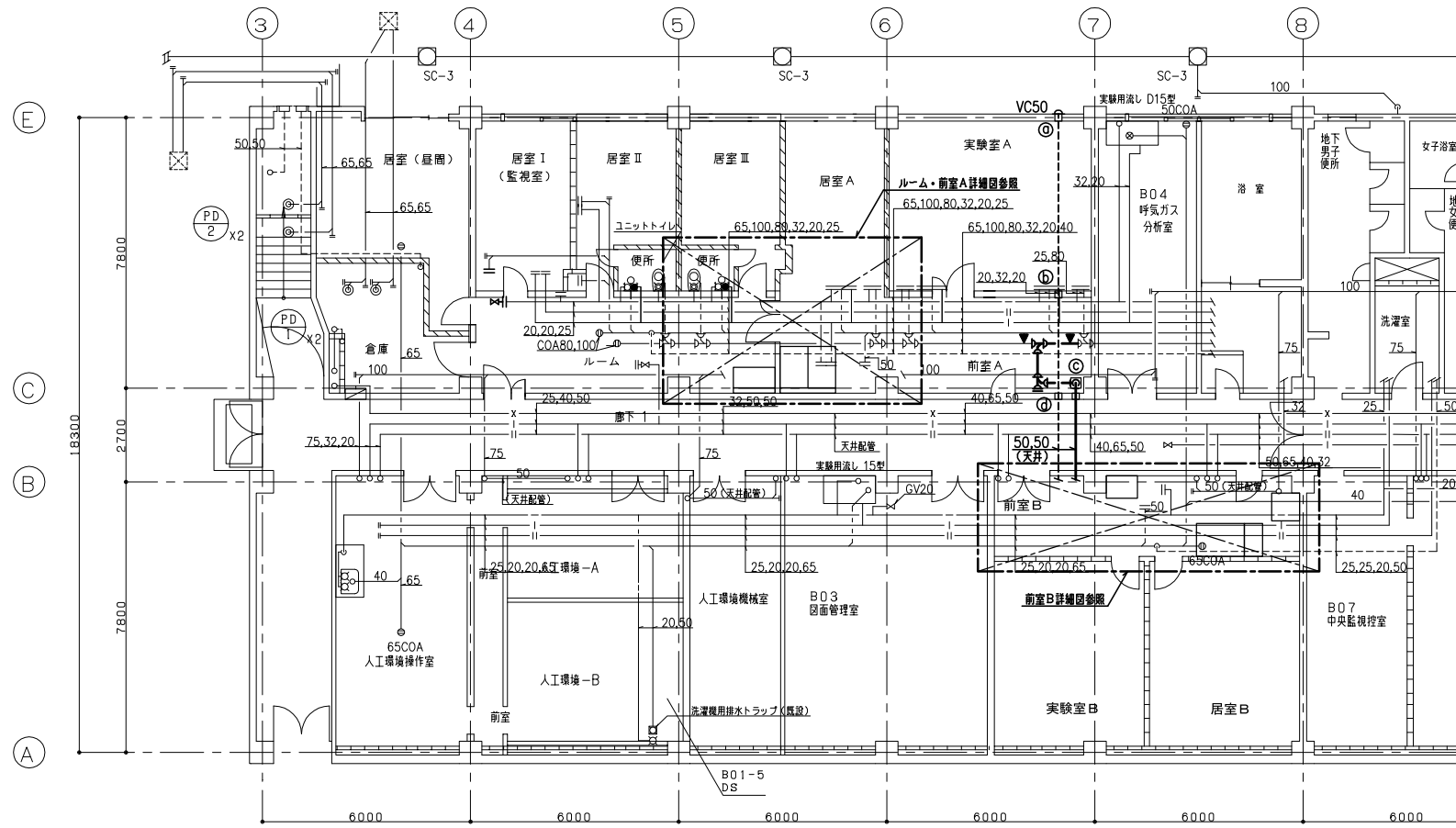
改修 研究本館 衛生設備 B1階平面図 S=1/100
