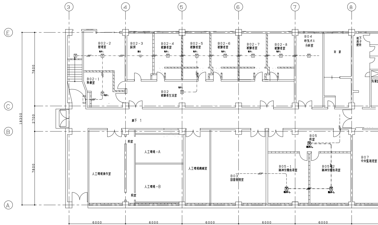
撤去 研究本館 電気設備 B1階自動火災報知設備平面図 S=1/100
