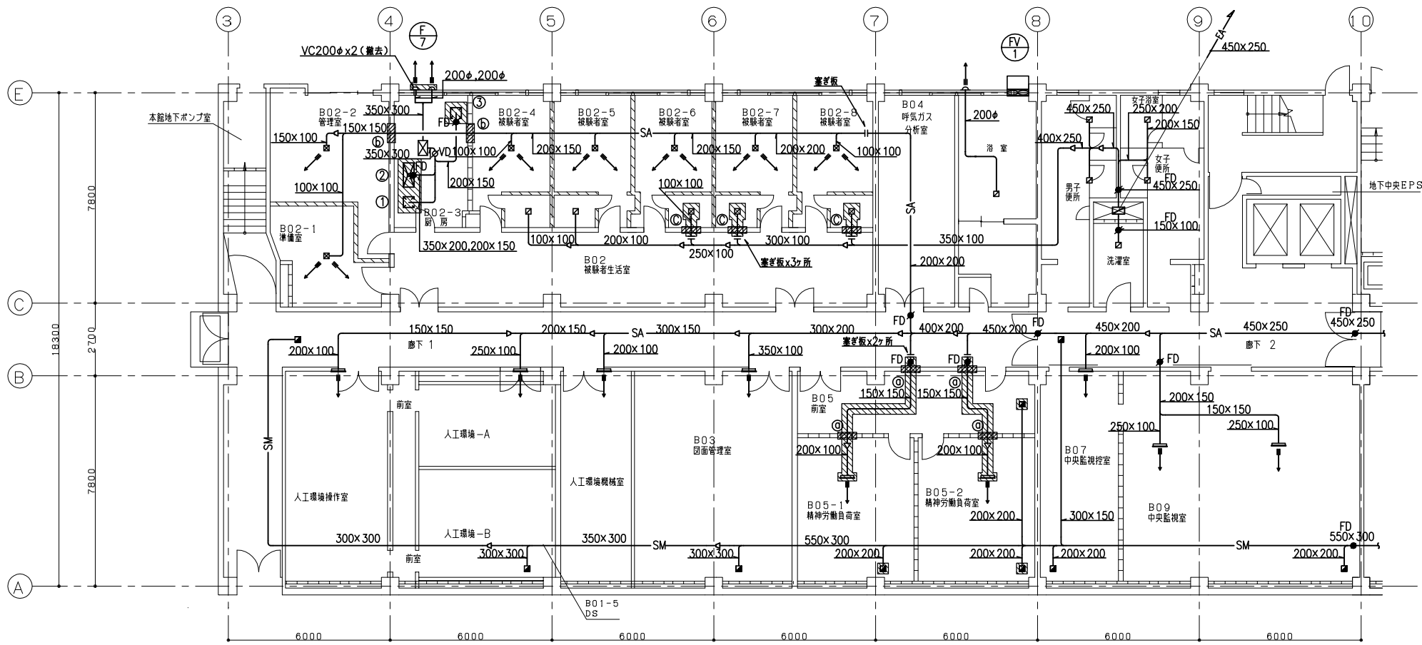
撤去 研究本館 空調設備 B1階ダクト平面図 S=1/100
