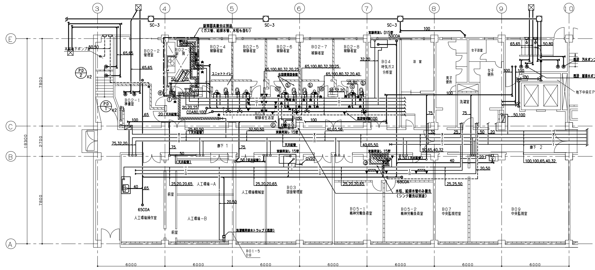
撤去 研究本館 衛生設備 B1階平面図 S=1/100
