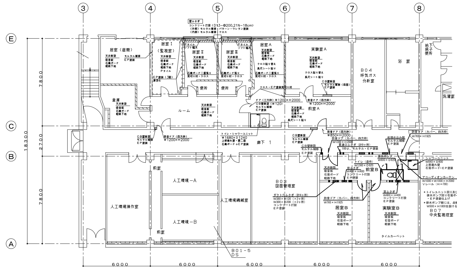
改設 研究本館棟 B1階平面図
