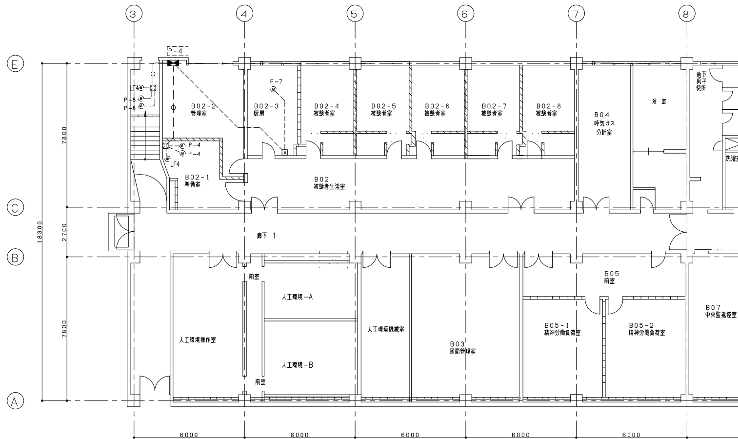
撤去 研究本館 電気設備 B1階空調電源設備平面図 S=1/100
