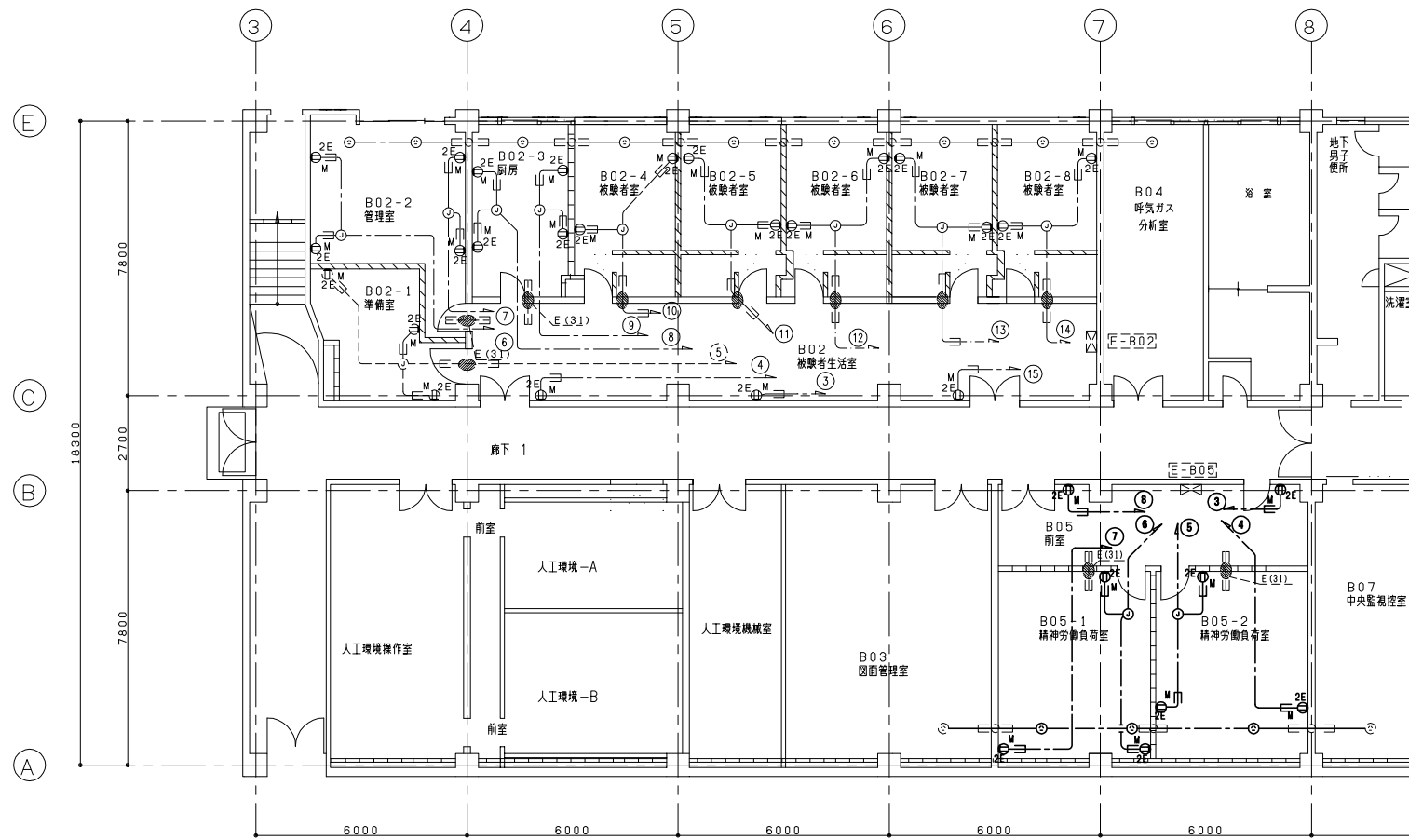
撤去 研究本館 電気設備 B1階コンセント設備平面図 S=1/100
