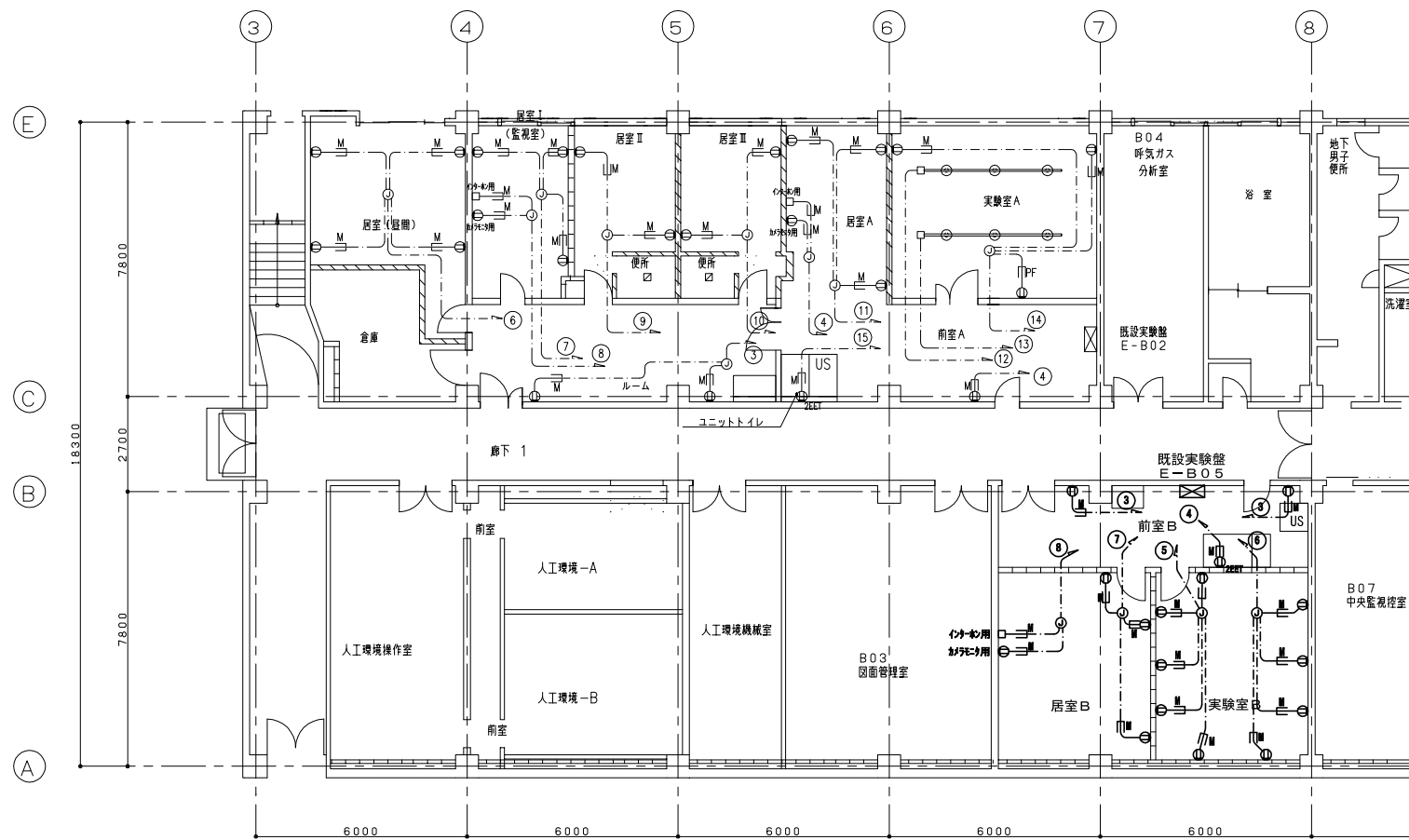
改修 研究本館 電気設備 B1階コンセント設備平面図 S=1/100
