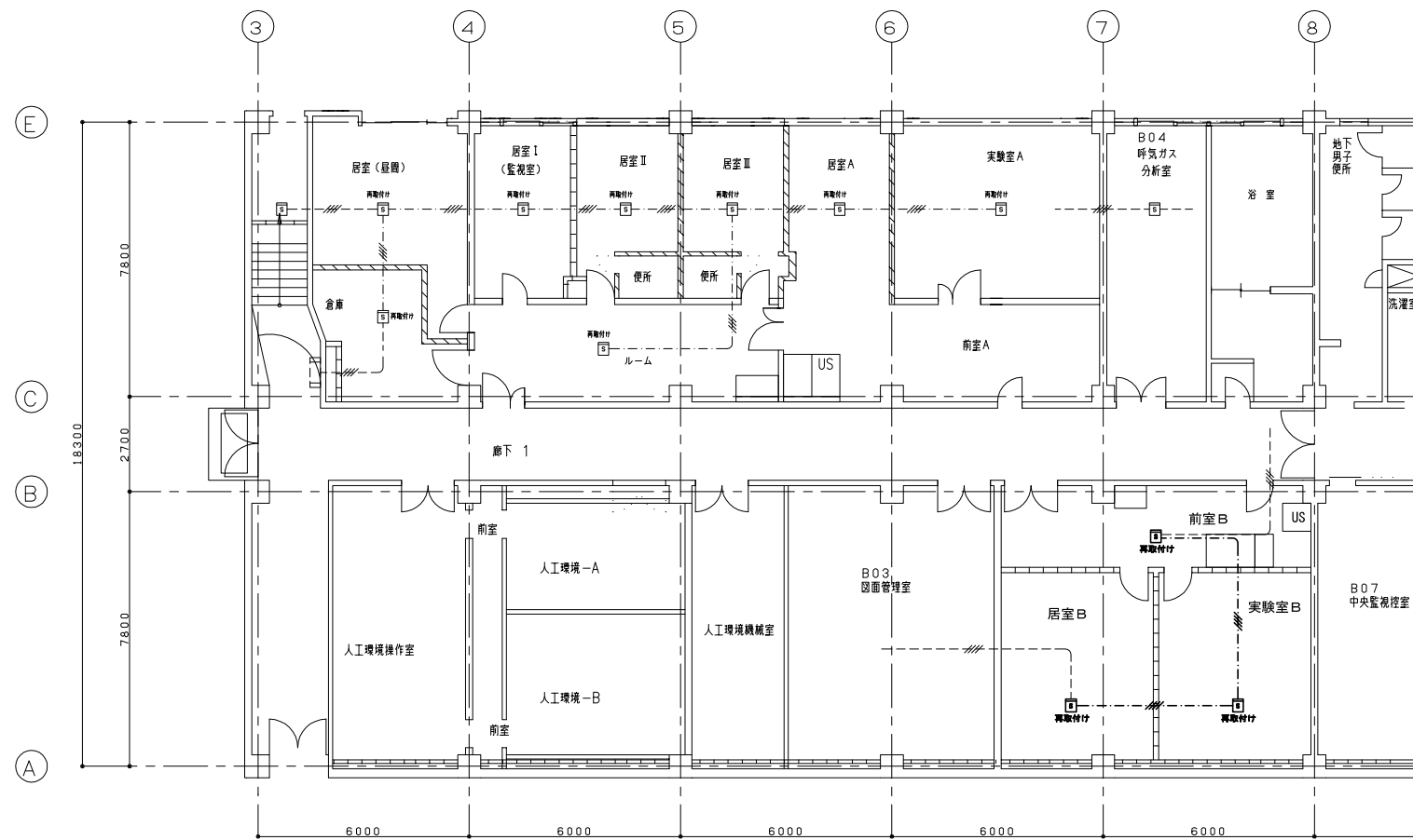
改修 研究本館 電気設備 B1階自動火災報知設備平面図 S=1/100
