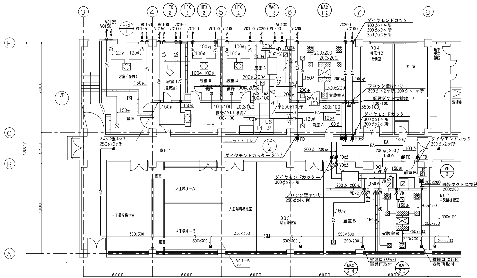
改設 研究本館 空調設備 B1階ダクト平面図 S=1/100
