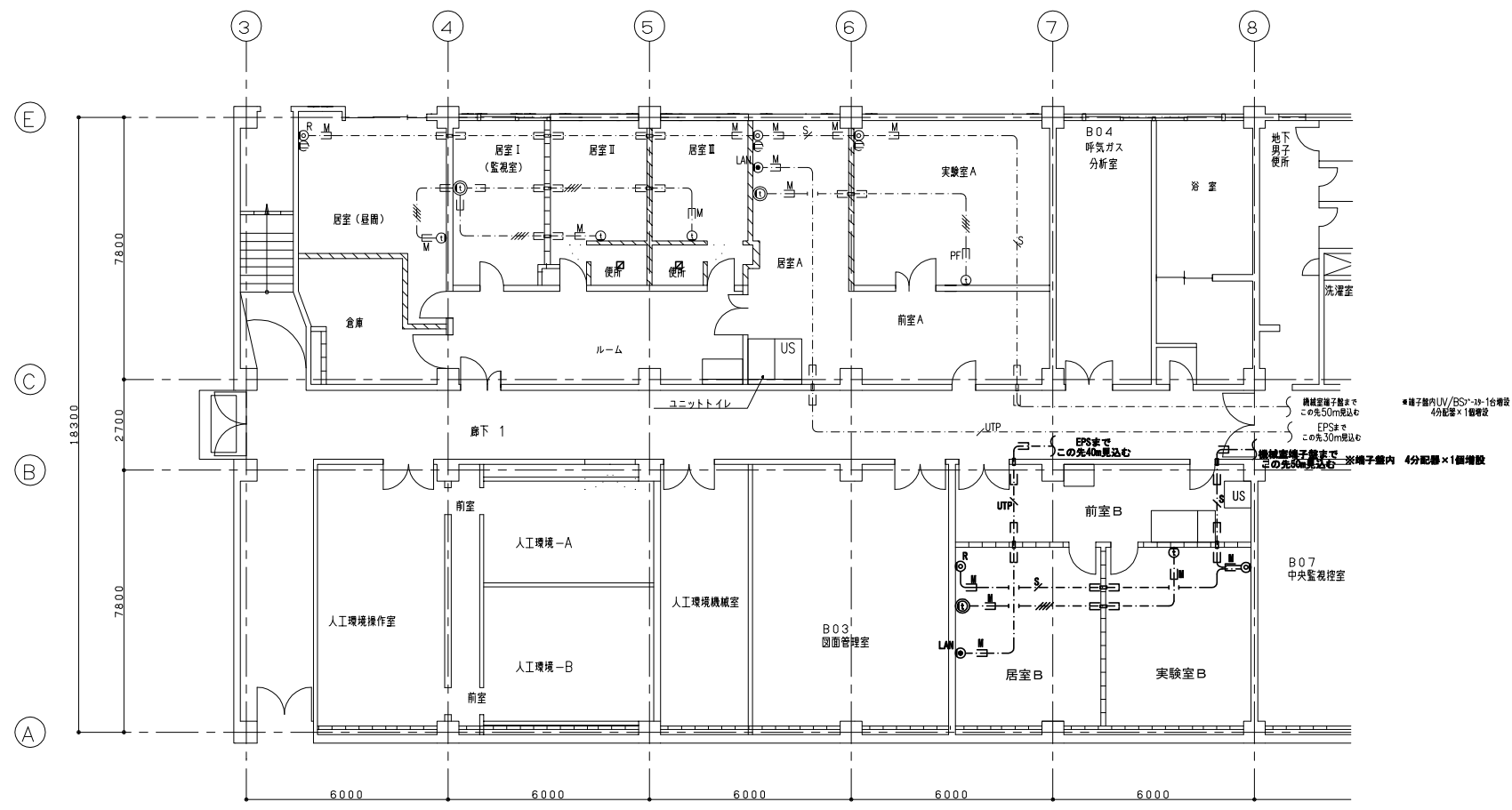
改修 研究本館 電気設備 B1階TV・LAN・インターホン設備平面図 S=1/100
