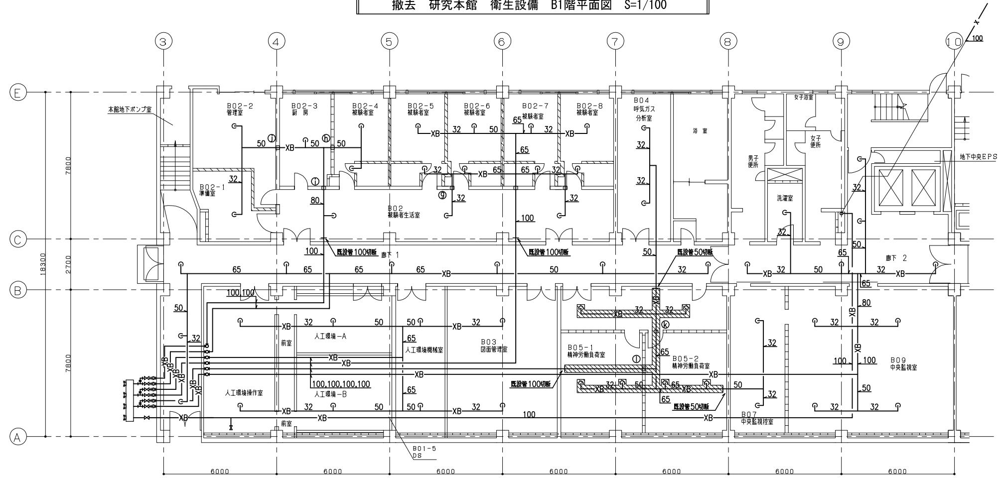
撤去 研究本館 消火設備 B1階平面図 S=1/100
