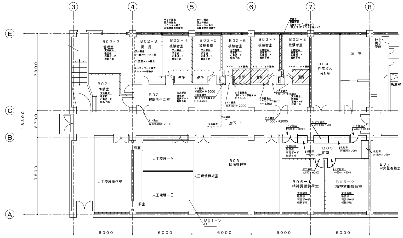
撤去 研究本館棟 B1階平面図
